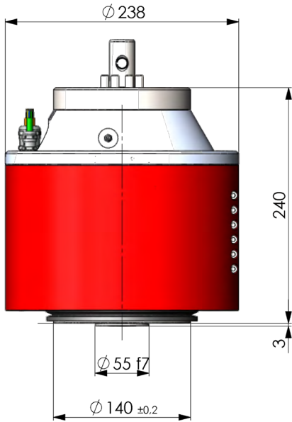
BV140 - Dimensions
